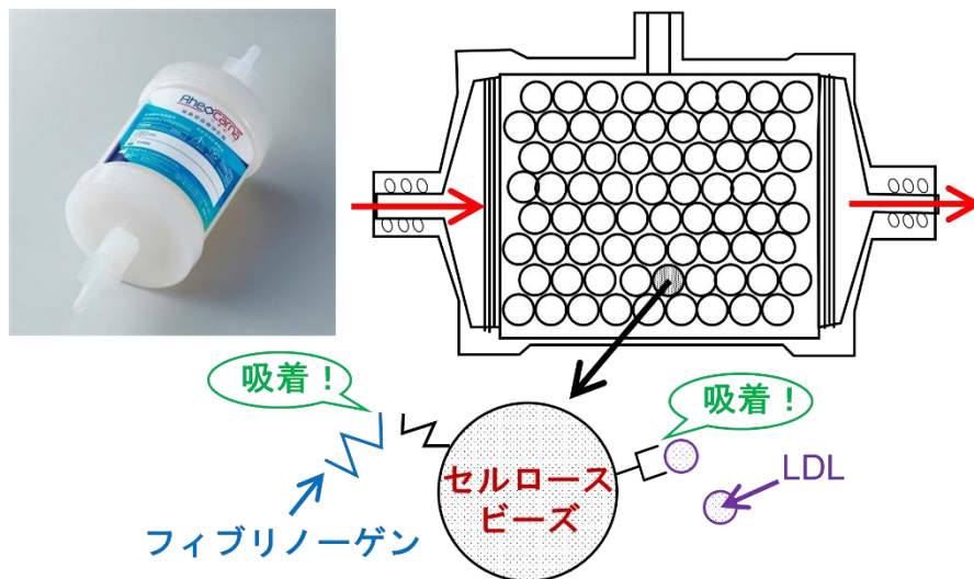
図 2. レオカーナによる LDL・フィブリンノーゲン吸着
